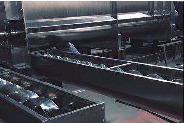
螺旋输送机装配制作中
