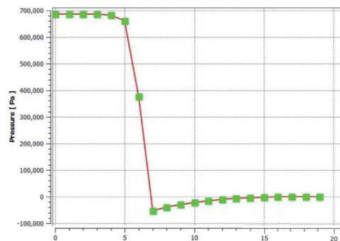
轴线上压力分布
