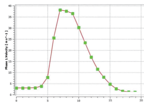
轴线上速度分布
